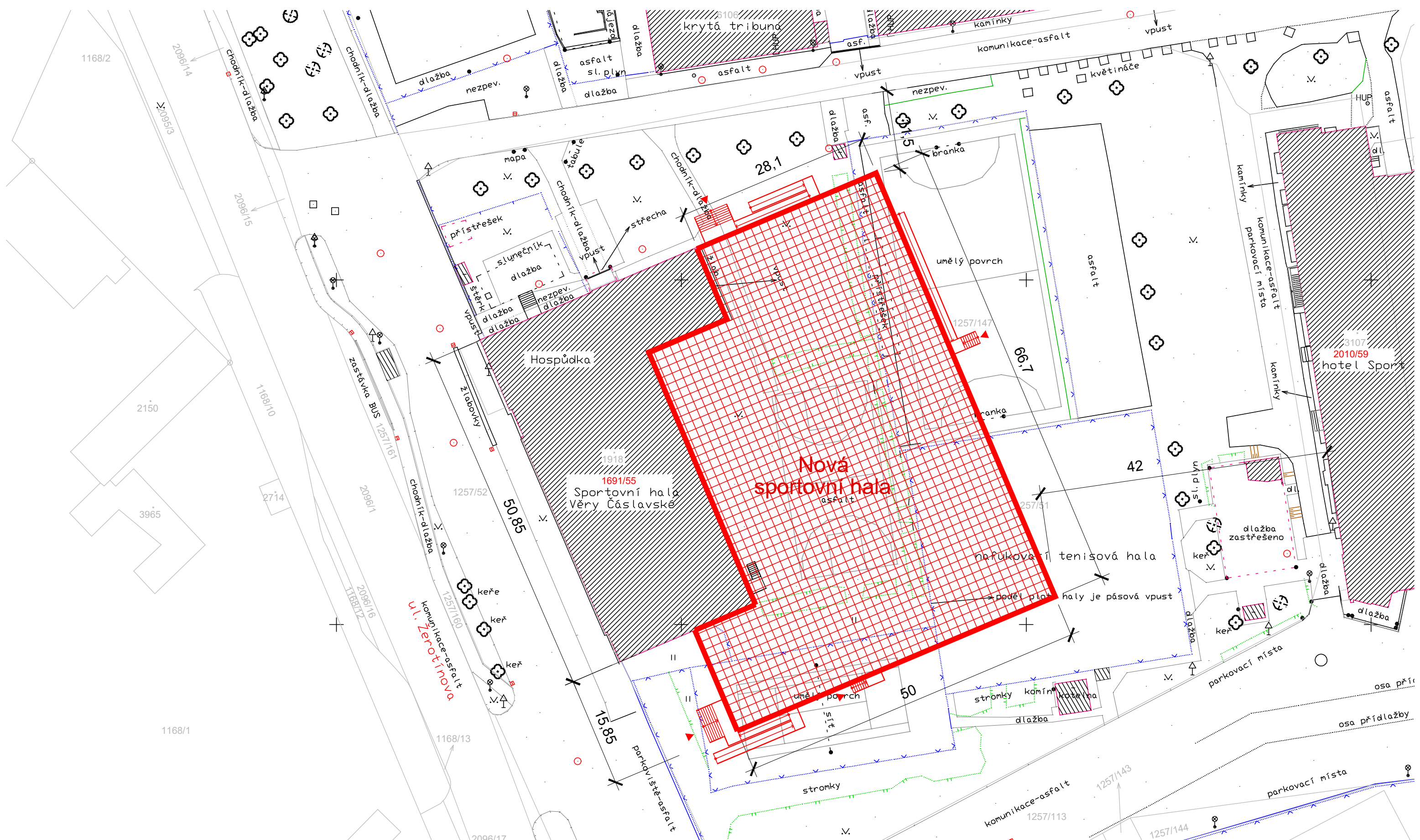
Sportovní hala pro míčové sporty v areálu Tyršova stadionu Šumperk Situace stavby haly M = 1:500
